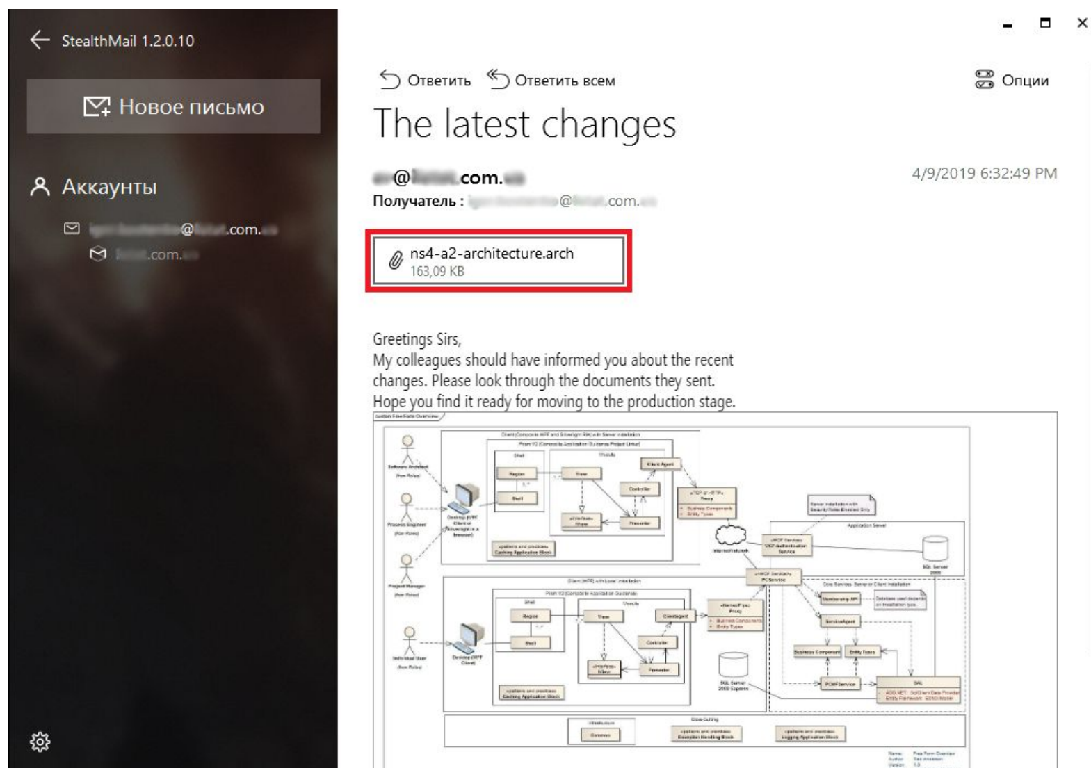
Рис.5.5 Вложения письма
