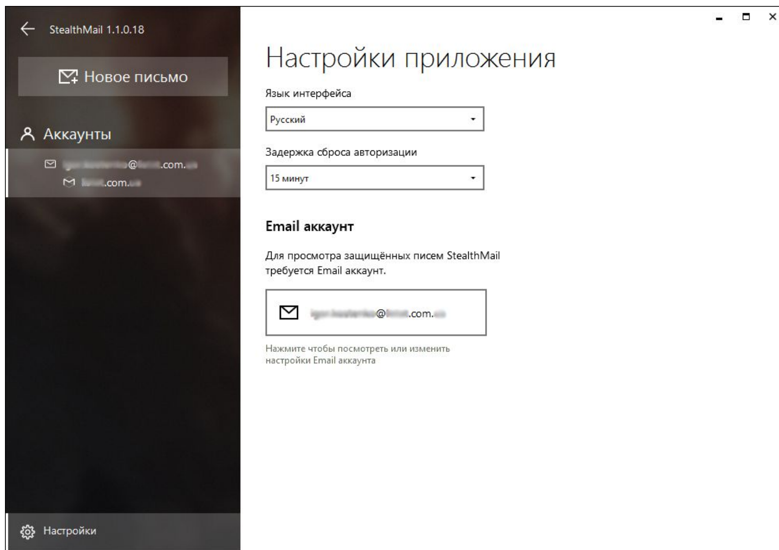
Рис.6 Меню Настройки
