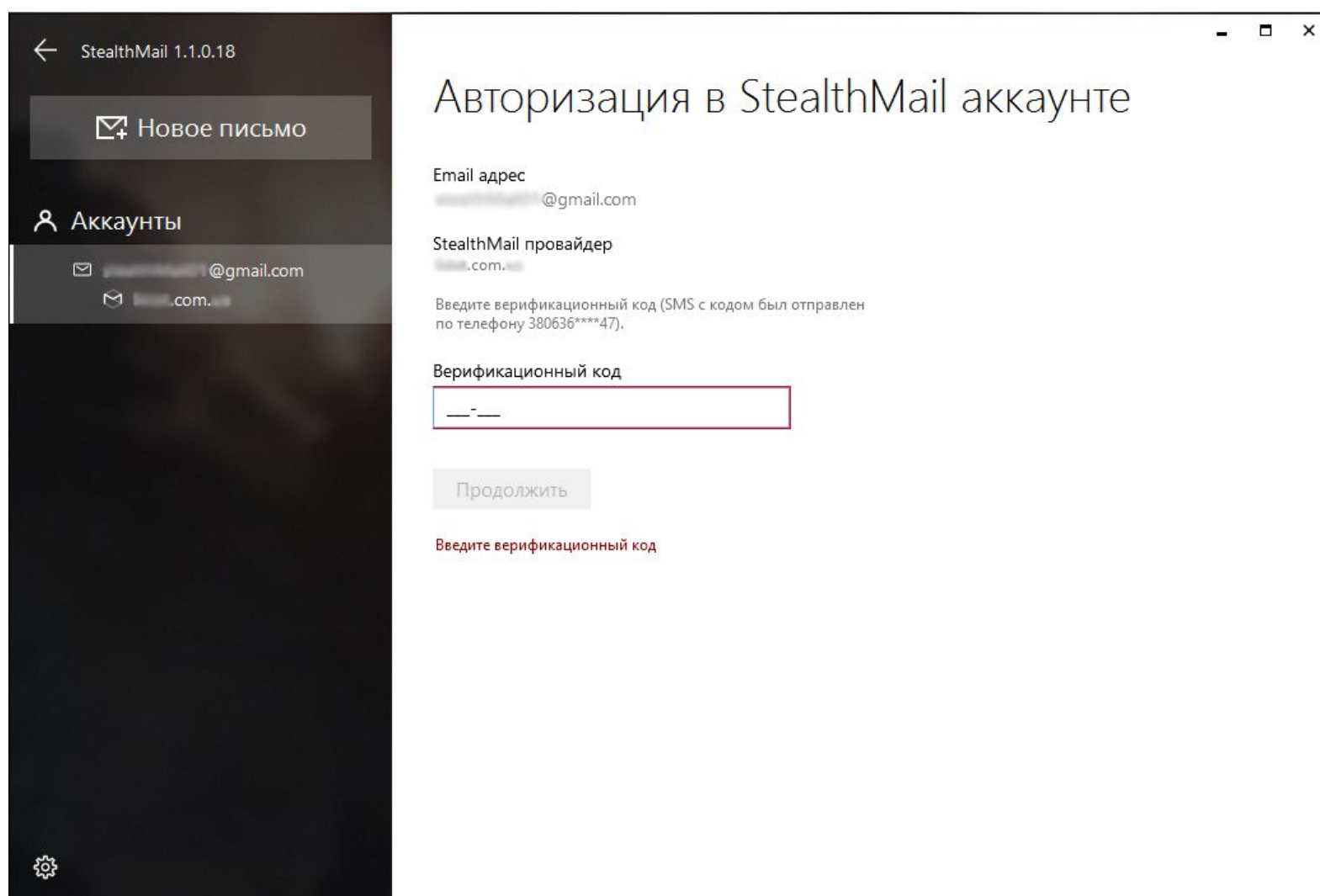
Рис.7.1-2 Восстановление пароля
